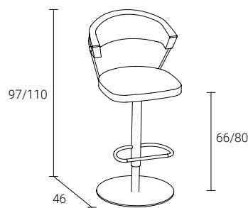
Great con seduta girevole regolabile in altezza Great with height- adjustable revolving seat
